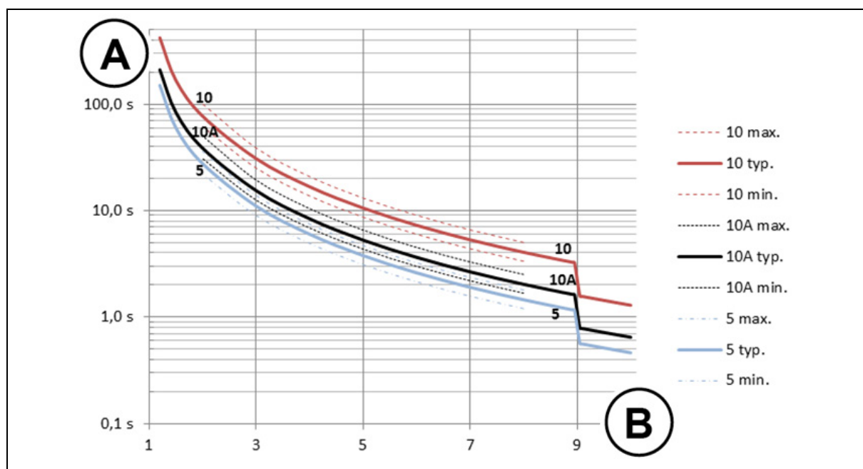
Figura 4: Curvas características de las clases de activación
