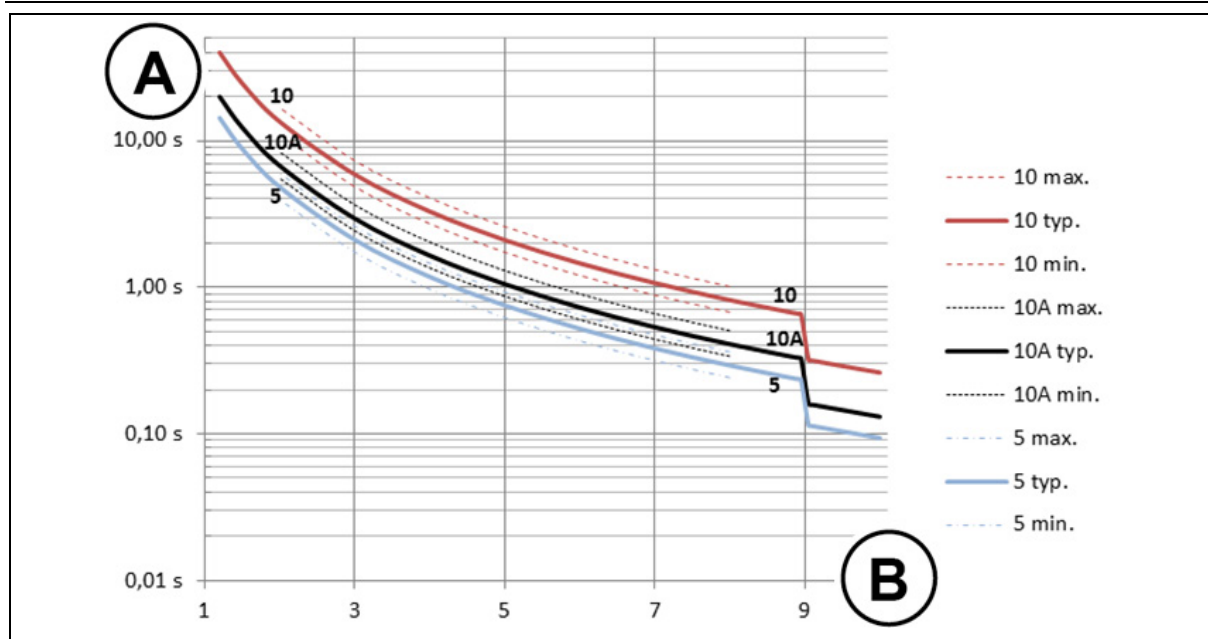
Figura 5: Tiempos de activación desde el estado funcionamiento en caliente (en caso de: I = I_{nom} de forma permanente.)
