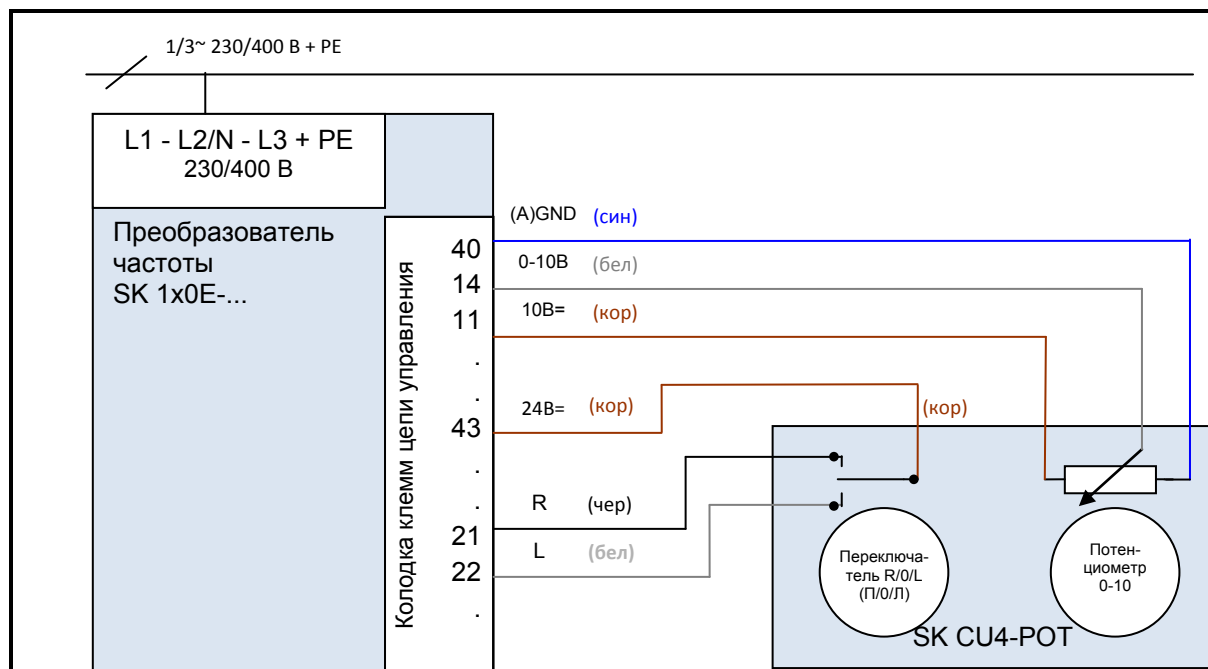
Рис. 13: Схема соединения SK CU4-POT, пример для SK 1x0E
