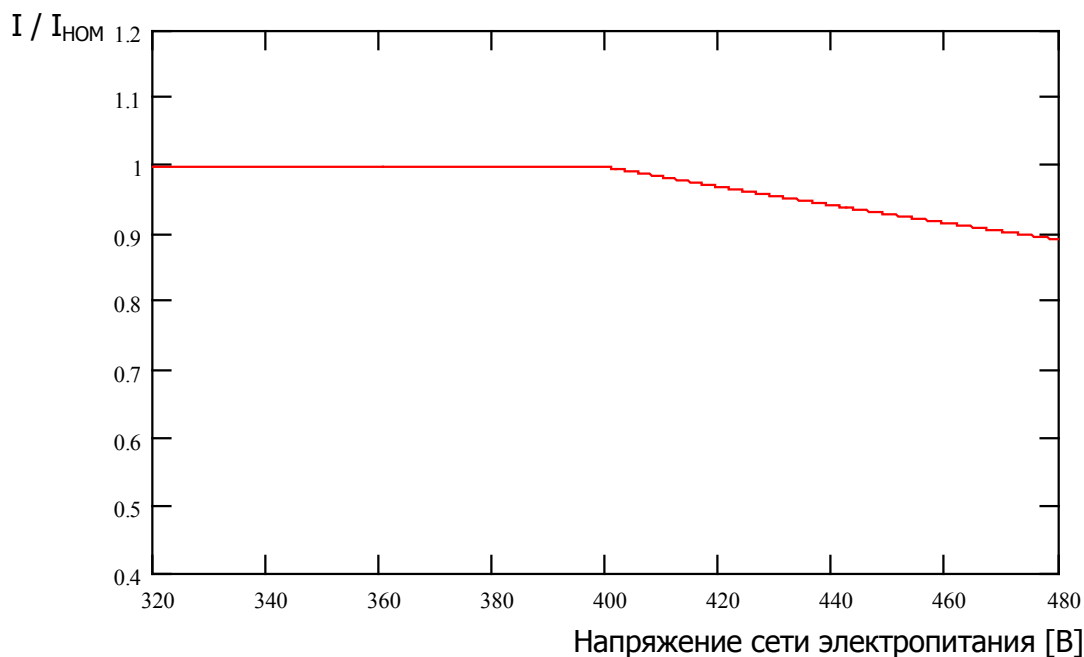
Рис. 19: Выходной ток в зависимости от сетевого напряжения
