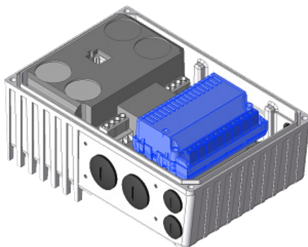
Рис. 1: Устройство со встроенным модулем SK CU4-...
