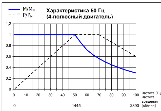
Рис. 21: Характеристика 50 Гц
