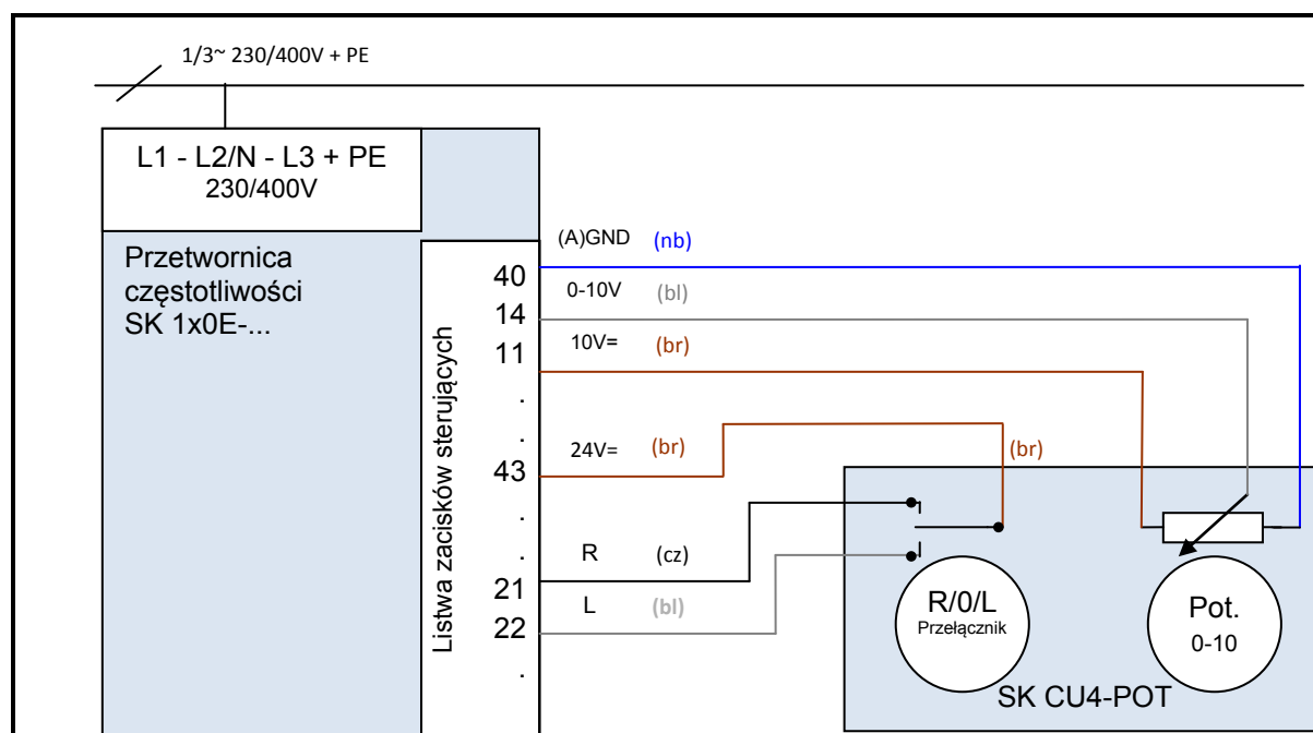
Rysunek 5: Schemat podłączeń SK CU4-POT, przykład SK 1x0E
