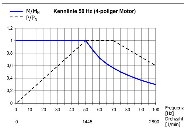
Abbildung 38: Kennlinie 50 Hz
