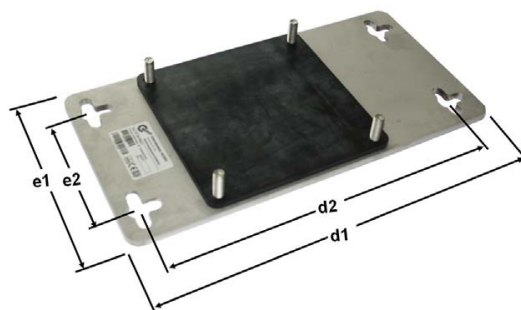
Abbildung 9: SK TIE4-WMK-3
