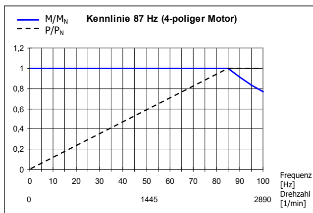
Abbildung 39: Kennlinie 87 Hz
