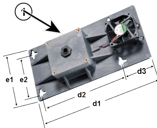
1 Einführung Lüfter-Anschlusskabel
