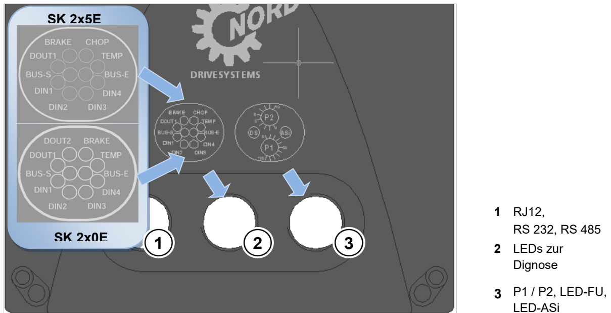
Abbildung 30: Diagnoseöffnungen SK 2x0E BG 4 bzw. SK 2x5E
