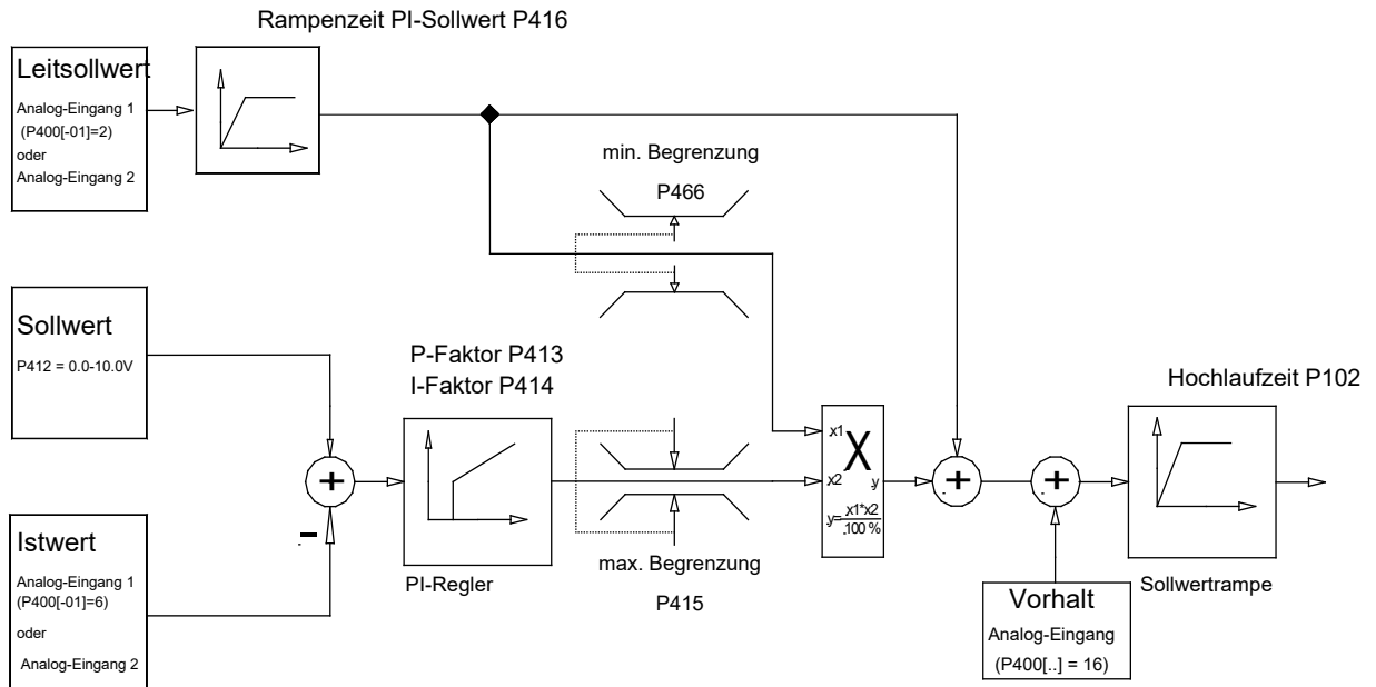
Abbildung 32: Ablaufdiagramm Prozessregler
