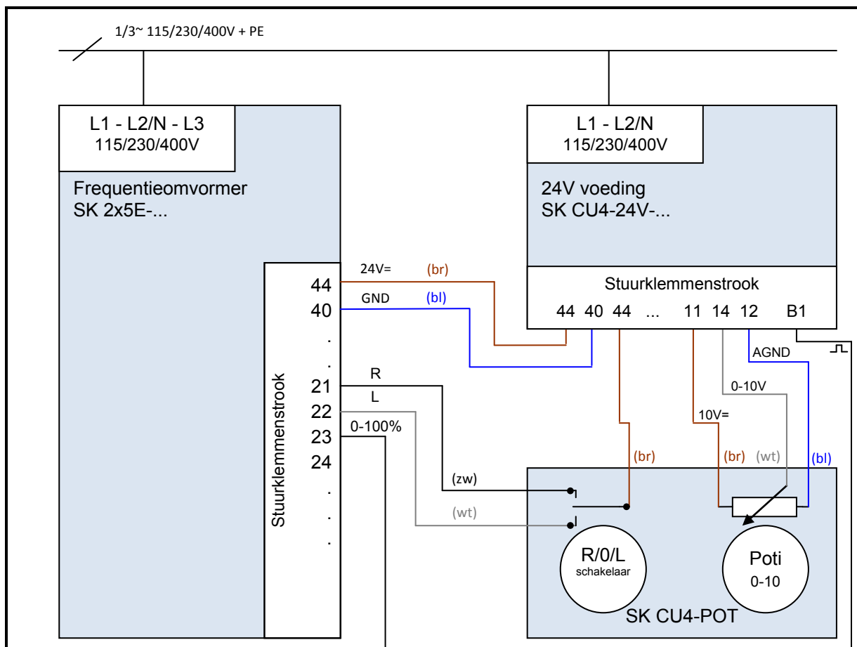
Afbeelding 10: Aansluitschema SK CU4-POT en parameterinstellingen, voorbeeld SK 2x5E
