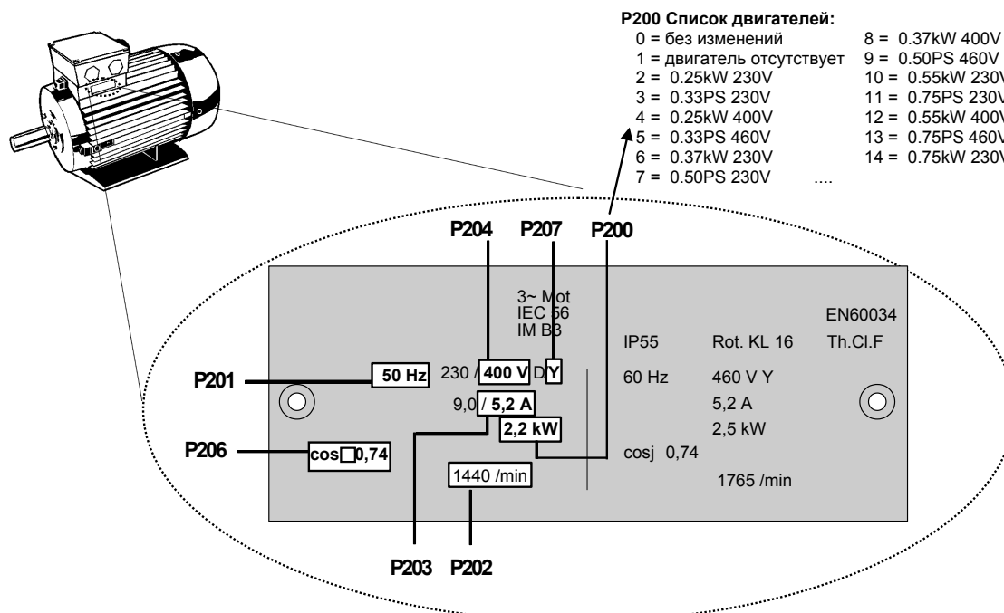
Рис. 13: Паспортная табличка двигателя
