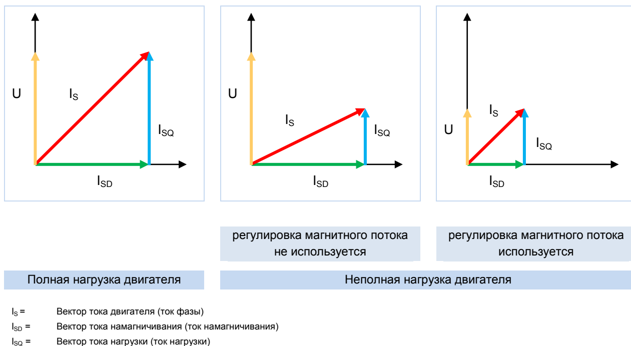
Рис. 19: Изменение энергоэффективности при использовании автоматической регулировки намагничивания
