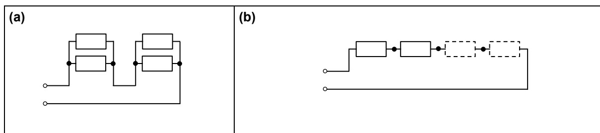
Рис. 6: Стандартные схемы подключения тормозных резисторов
