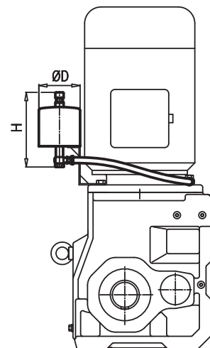
Kúpkeres hajtómű
