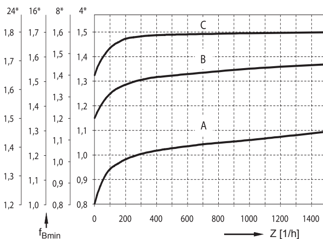
1. ábra: Minimális üzemi tényező f_{Bmin}
