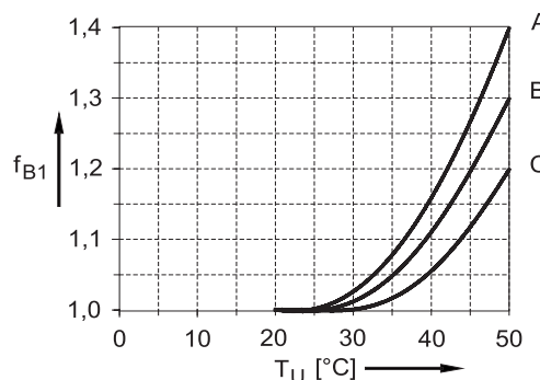
2. ábra: Üzemi tényező f_{B1}
