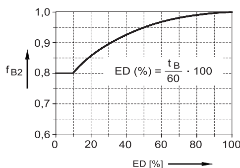
3. ábra: Üzemi tényező f_{B2} ED = bekapcsolási idő t_B = terhelési idő perc/óra
