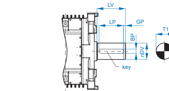
アウトプットソリッドシャフト
