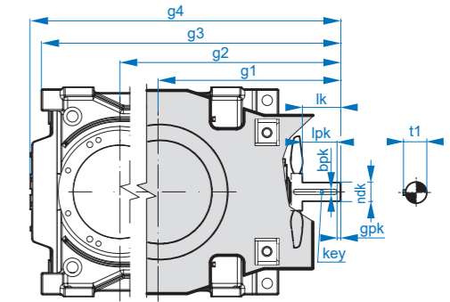
ドライブソリッドシャフト
