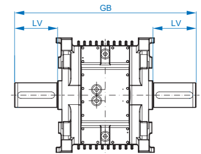
ダブルアウトプットソリッドシャフト
