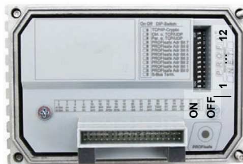
Werkseinstellung DIP-Schalter: OFF
